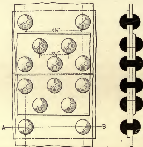
FIG. 44.—DOUBLE-WELT BUTT-JOINT.
